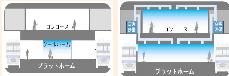
改修前(クールルームのみ冷房)
