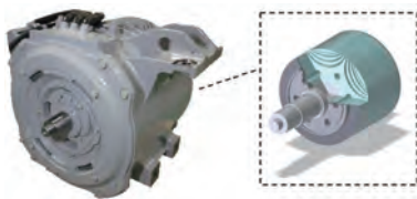
同期リラクタン্সモーター
