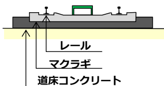
(軌道工事の標準断面図)
