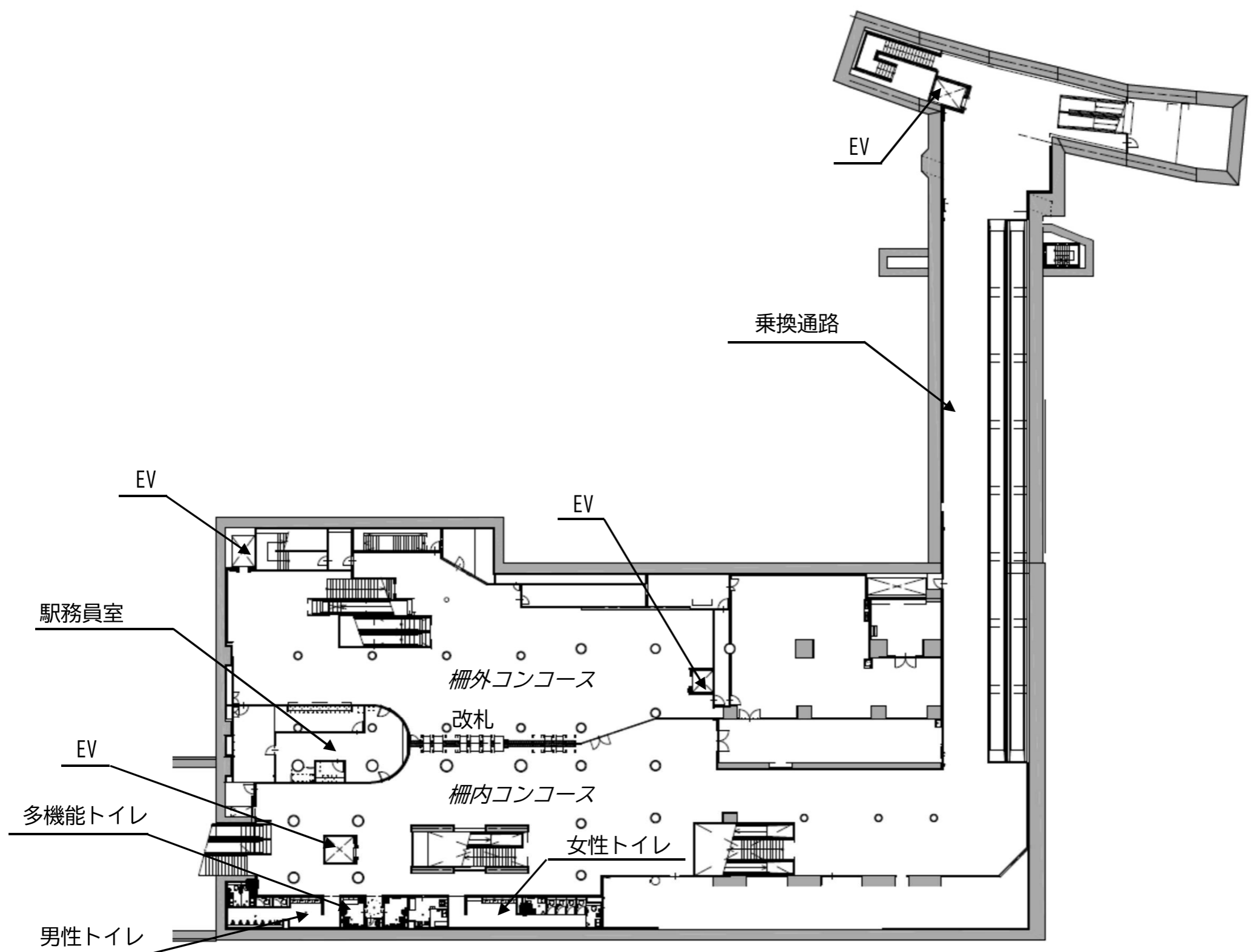
別添資料5：七隈線博多駅平面図
