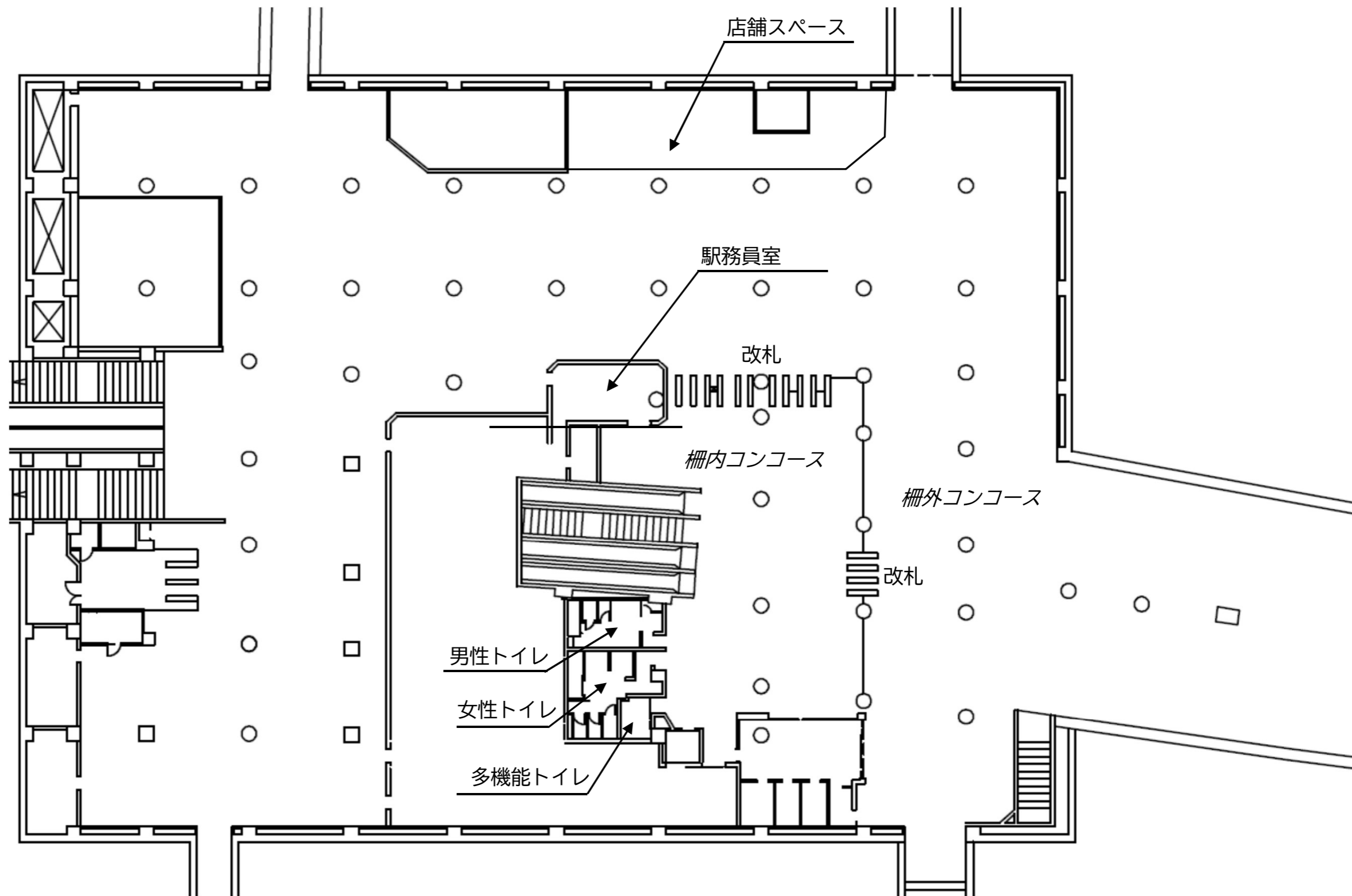
別添資料3：空港線博多駅（筑紫口）平面図
