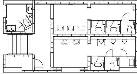
トイレ平面レイアウト
